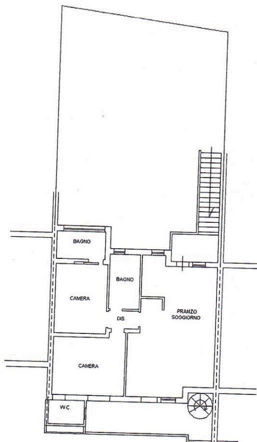
PIANTA PIANO PRIMO h = 2,80
